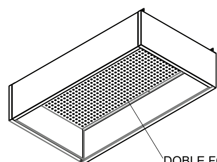
DOBLE FONDO EN TOLDO INTERIOR MULTIPERFORADO
