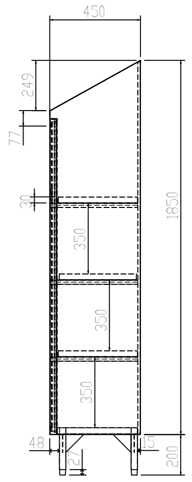
VISTA LATERAL
