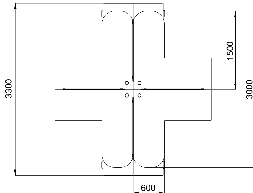
Vista Superior
